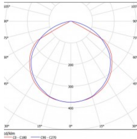
График КСС
